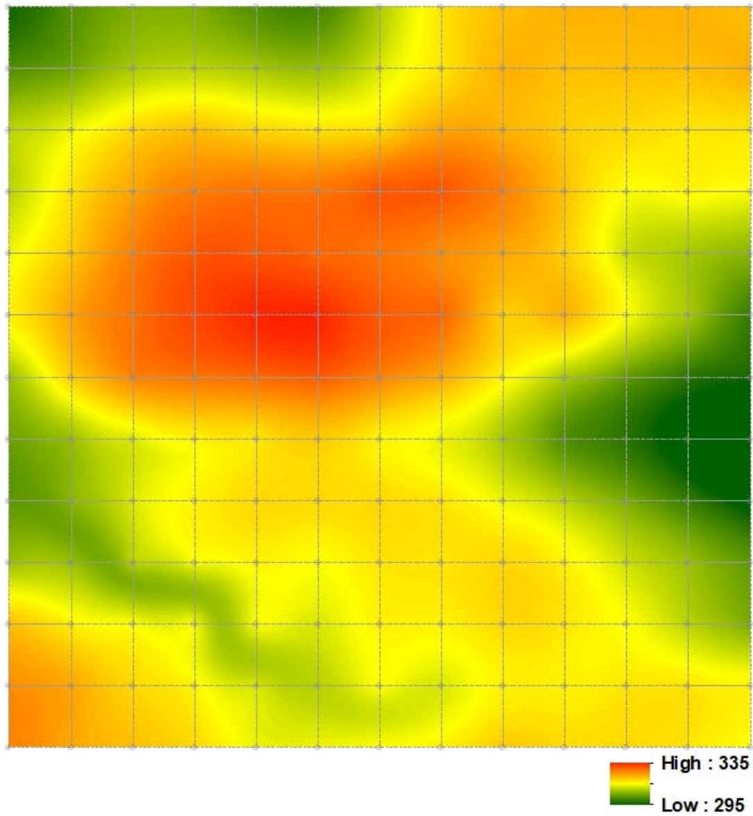
ภาพที่ 8 ระดับสูงต่ำของภูมิประเทศในแปลงตัวอย่าง
