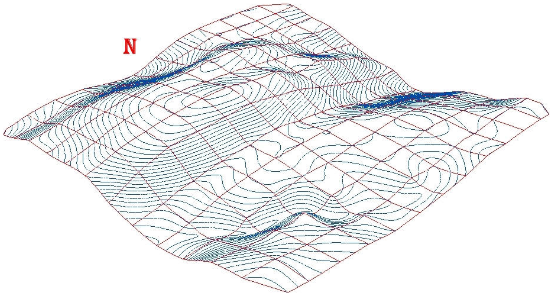
ภาพที่ 10 แบบจำลอง 3 มิติ เส้นชั้นระดับความสูงบริเวณแปลงตัวอย่าง
