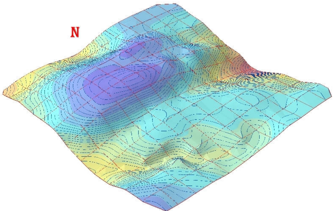
ภาพที่ 11 แบบจำลอง 3 มิติ สภาพภูมิประเทศบริเวณแปลงตัวอย่าง
