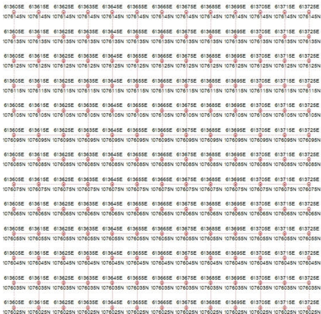
ภาพที่ 5 พิกัดภูมิศาสตร์ในระบบ UTM ของหมุดในแต่ละแปลงย่อย
